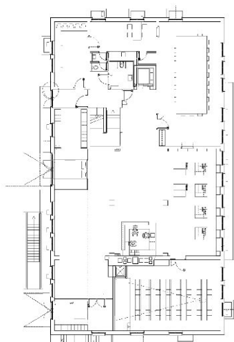
Erdgeschoß
