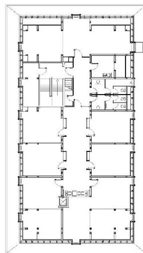
Obergeschoß
